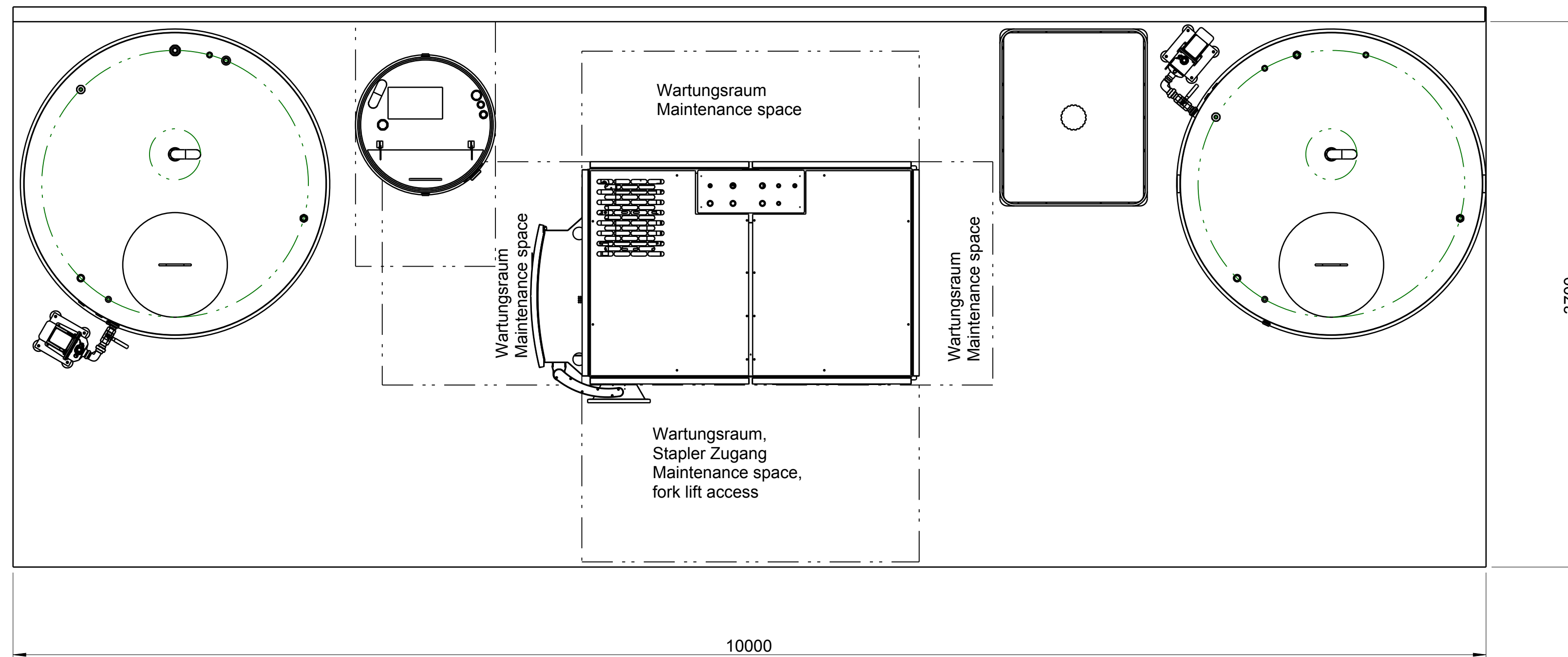
Draufsicht Top view
