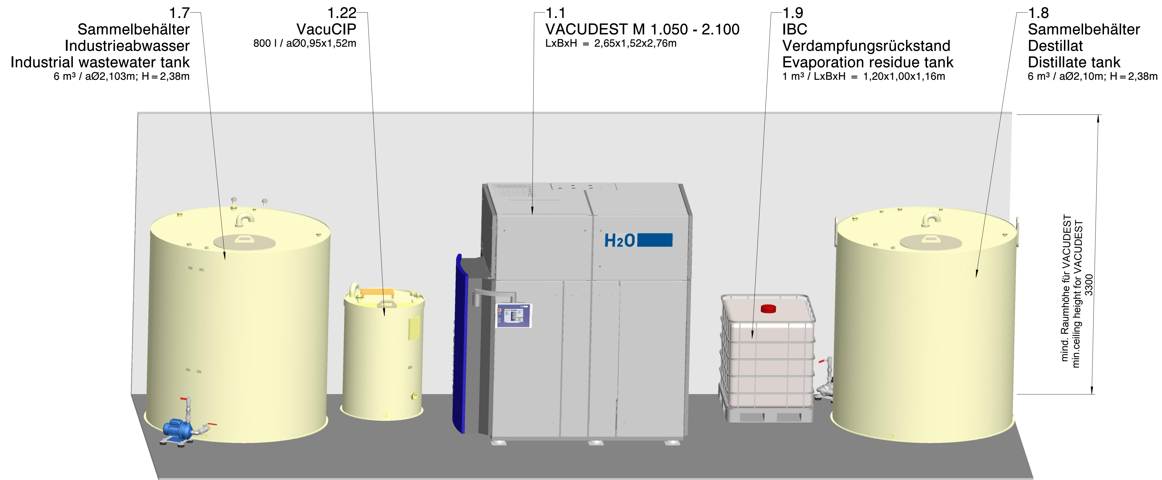
Vorderansicht Front view
